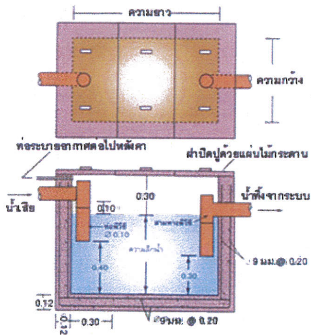
บ่อดักไขมันแบบสร้างในที่สำหรับอาคารขนาดใหญ่อาศัย
